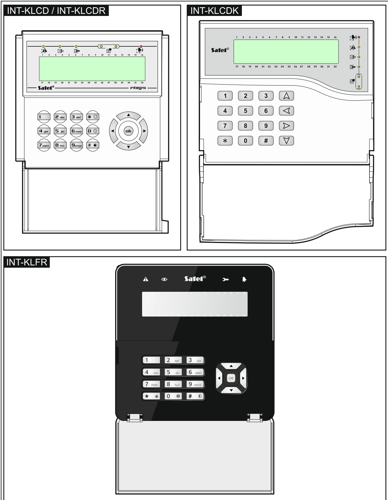
Abb. 1. Bedienteile mit Klappen.
