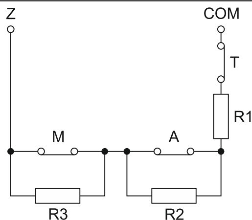
Abb. 4. Nummerierung der Abschlusswiderstände. T – Sabotage. A – Alarm. M – Abdeckung. Bei den Konfigurationen EOL und 2EOL hat der Wert des Widerstandes R3 keine
